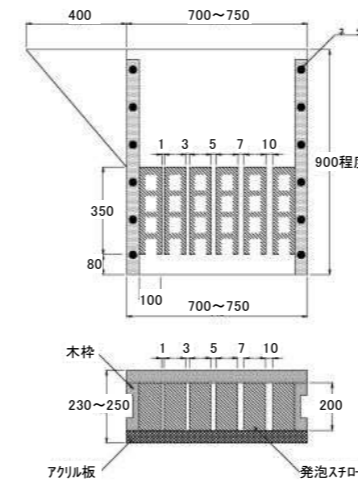
図-2 試験装置(非漏出性試験)
