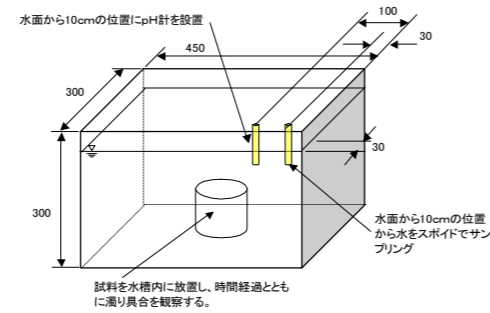
図-3 試験装置(水中分離抵抗性試験)
