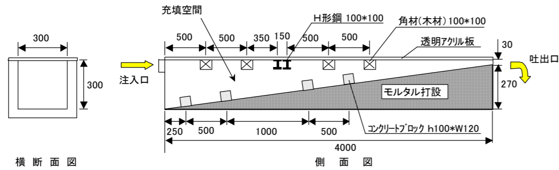
図-1 試験装置(充填性試験)
