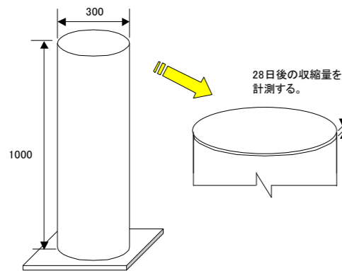
図-4 試験装置(非収縮性試験)
