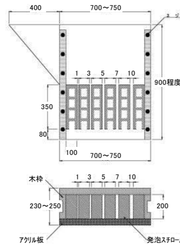
図-2 試験装置(非逸走性試験)
