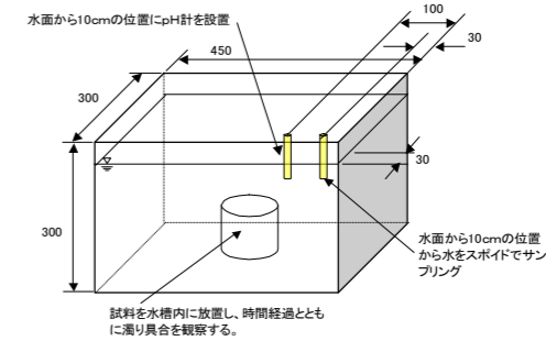
図-3 試験装置(水中分離抵抗性試験)
